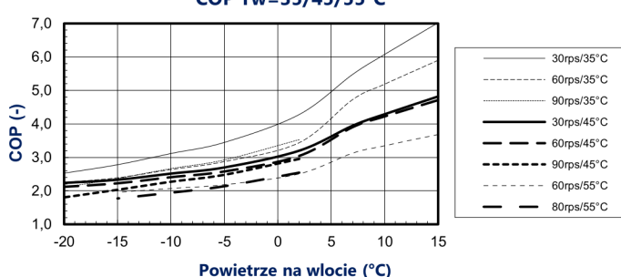
COP T_w=35/45/55^{\circ}C
